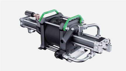
单驱双级气动气体增压器
