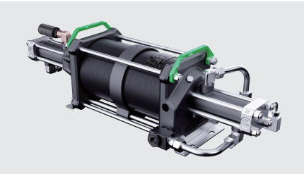
双驱双级气动气体增压器
