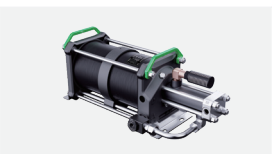
双驱单作用 双驱动活塞，每个工作循环实现一次增压，较相同压力比的单驱单作用流量更大，压缩空气能耗也更高。
